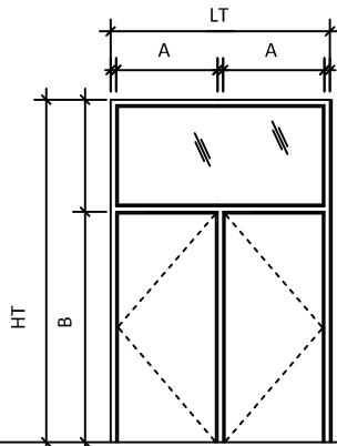
Élévation 7a
