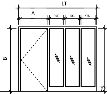
Élévation 36
