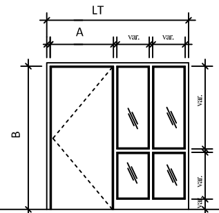
Élévation 27
