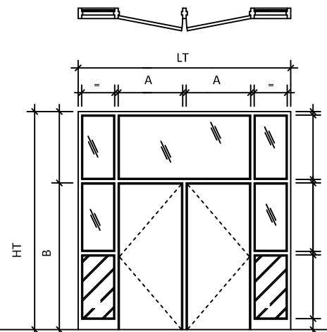
Élévation 14a
