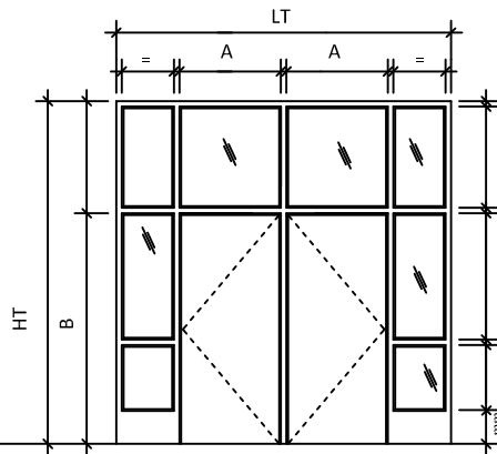
Élévation 81
