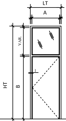
Élévation 6
