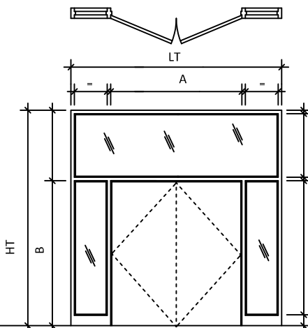
Élévation 14
