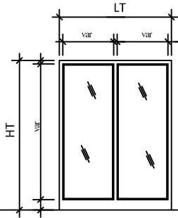
Élévation 64
