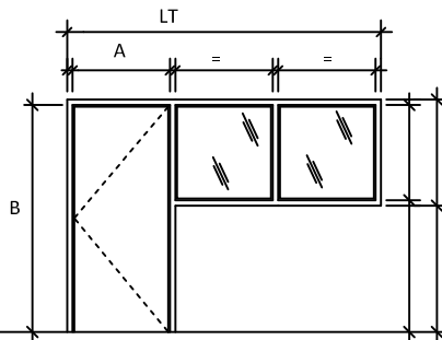
Élévation 10
