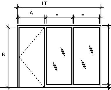
Élévation 35
