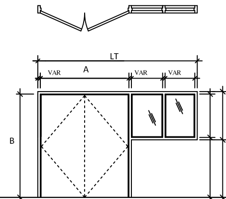
Élévation 23
