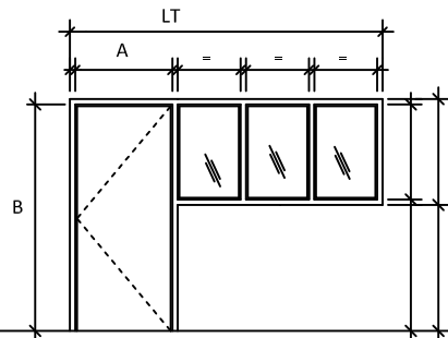
Élévation 20
