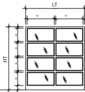
Élévation 56b
