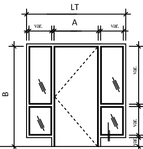
Élévation 25
