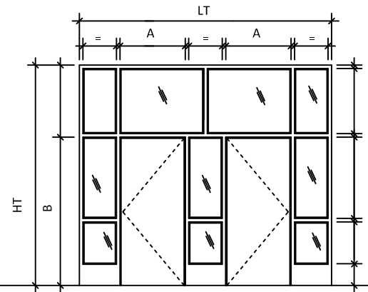
Élévation 86
