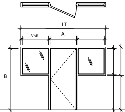
Élévation 13
