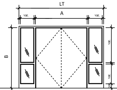
Élévation 31
