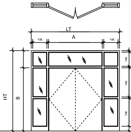
Élévation 49
