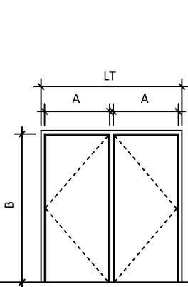
Élévation 3
