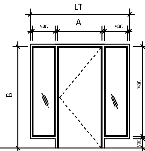
Élévation 33
