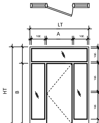
Élévation 47
