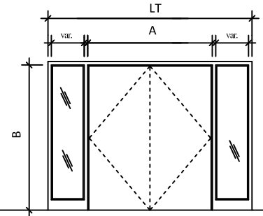
Élévation 37
