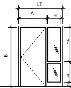
Élévation 26a
