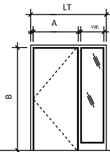
Élévation 11
