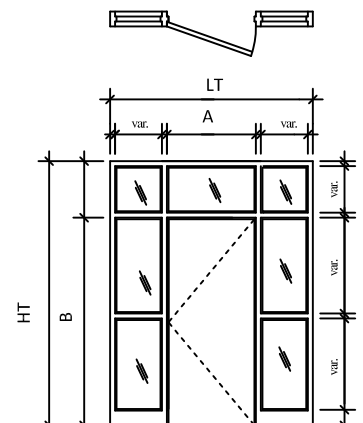
Élévation 48
