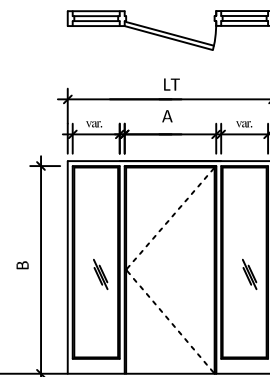
Élévation 12
