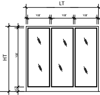
Élévation 65
