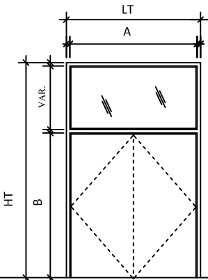
Élévation 7
