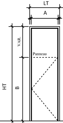
Élévation 4
