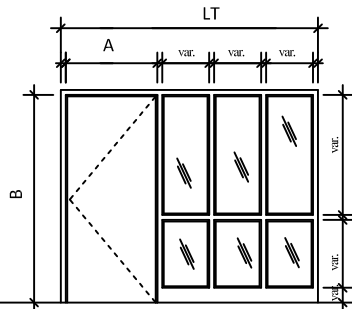
Élévation 28
