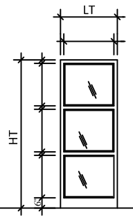
Élévation 55
