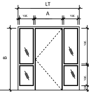
Élévation 30
