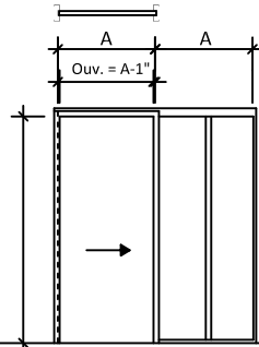
Élévation 1P
