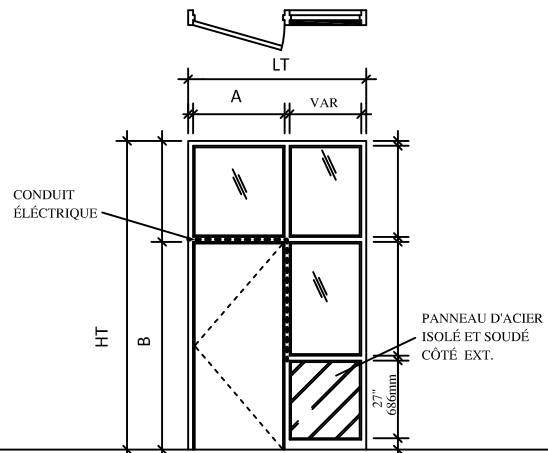
Élévation 8
