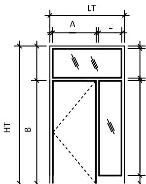
Élévation 19
