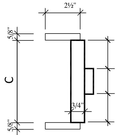
PROFIL B6
