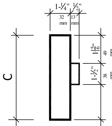
PROFIL B8
